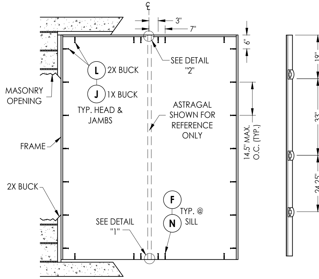
ASTRAGAL
